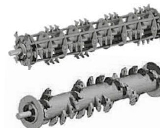
ROTOR FACAS HARDOX
